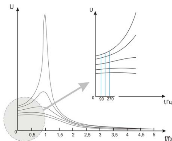
Рис. 1. Спектр затухающего синусоидального импульса. При увеличении \alpha он становится плоским. Спектр периодической последовательности импульсов на рисунке для f=90 Гц показан на фрагменте
