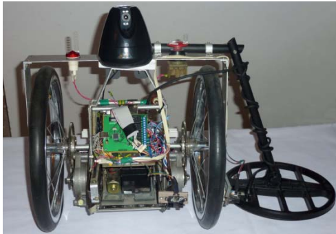
Рис. 1. Одноосный РС
