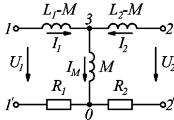
Рис. 4. Т-образная схема замещения трансформатора
